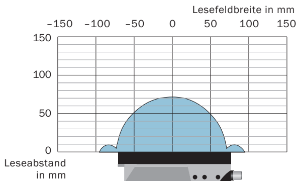
Lesefelddiagramm RFH62x
