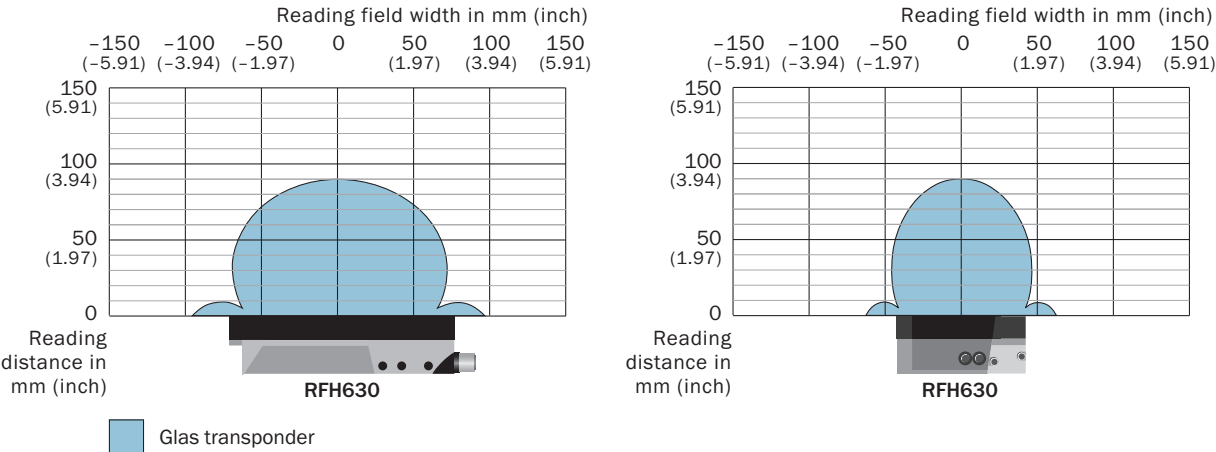
Диаграмма поля считывания RFH63x
