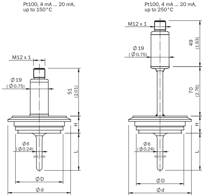
Rysunek wymiarowy
