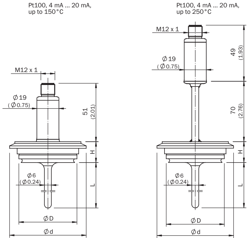
Rysunek wymiarowy
