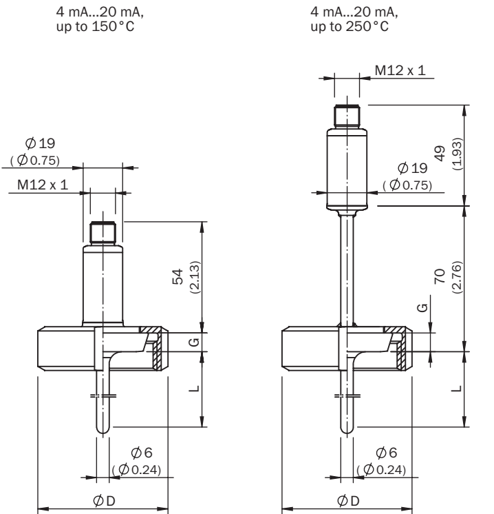
Rysunek wymiarowy
