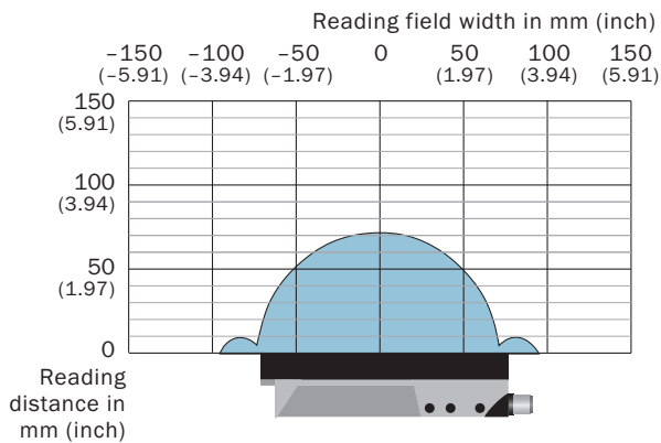
Wykres pola odczytu RFH63x
