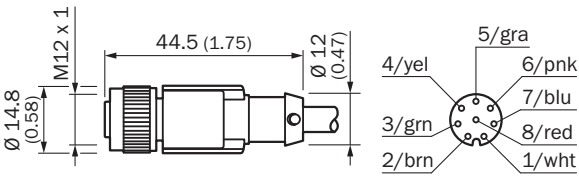
Rysunek wymiarowy (Wymiary w mm)
