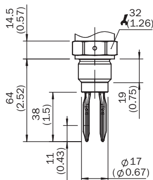
Габаритный чертеж корпуса
