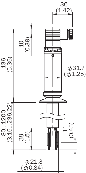
Габаритный чертеж
