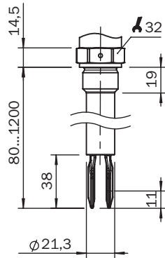
Maßzeichnung Gehäuse
