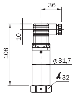
Maßzeichnung Gehäuse
