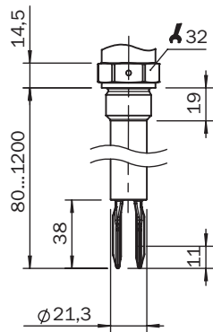
Maßzeichnung Gehäuse
