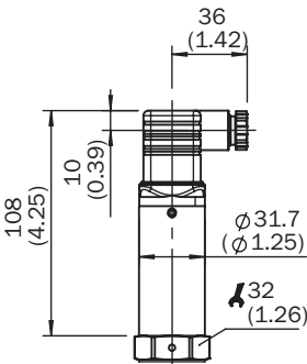
Габаритный чертёж корпуса
