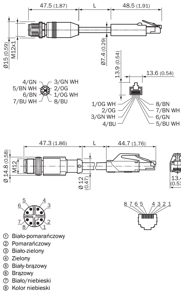
Rysunek wymiarowy (Wymiary w mm)
