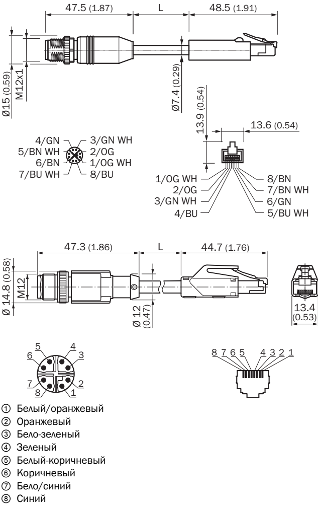
Габаритный чертеж (Размеры, мм)
