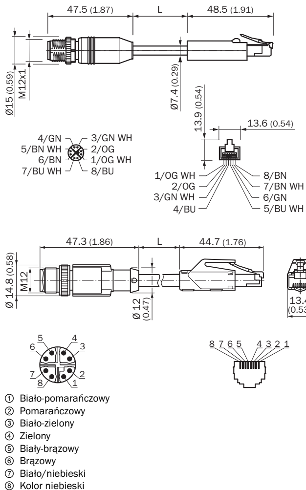
Rysunek wymiarowy (Wymiary w mm)
