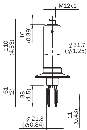
Rysunek wymiarowy
