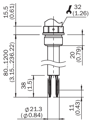
Габаритный чертеж корпуса
