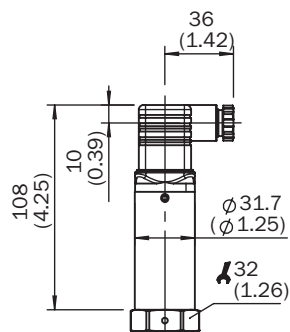
Габаритный чертеж корпуса
