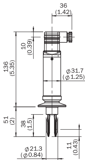
Rysunek wymiarowy
