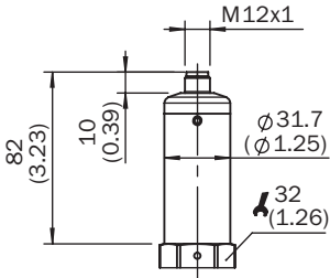
Габаритный чертёж корпуса
