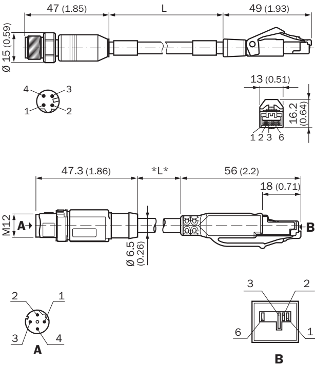
Rysunek wymiarowy (Wymiary w mm)
