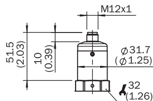
Rysunek wymiarowy: obudowa
