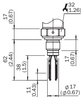
Rysunek wymiarowy: obudowa
