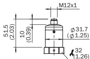
Габаритный чертеж корпуса
