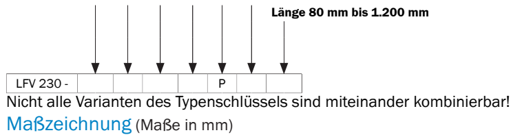
Maßzeichnung Prozessanschluss
