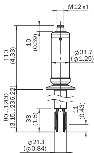
Rysunek wymiarowy
