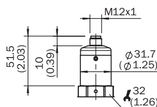
Rysunek wymiarowy: obudowa
