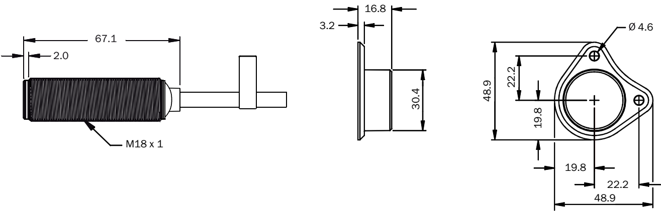
Rysunek wymiarowy (Wymiary w mm)
