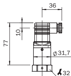
Maßzeichnung Gehäuse
