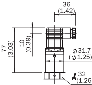
Габаритный чертеж корпуса
