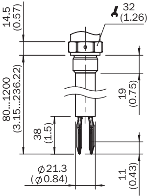
Габаритный чертёж корпуса
