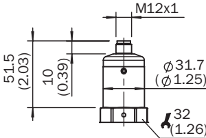
Габаритный чертёж корпуса
