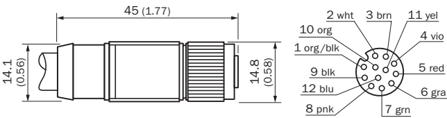
Rysunek wymiarowy (Wymiary w mm)
