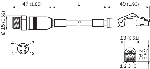
Габаритный чертеж (Размеры, мм)
