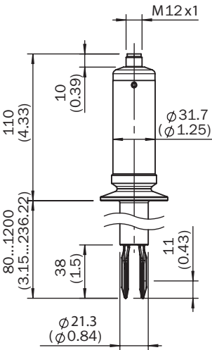
Габаритный чертеж корпуса
