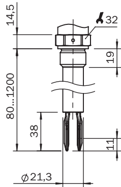
Maßzeichnung Gehäuse
