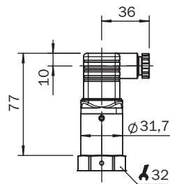
Maßzeichnung Gehäuse
