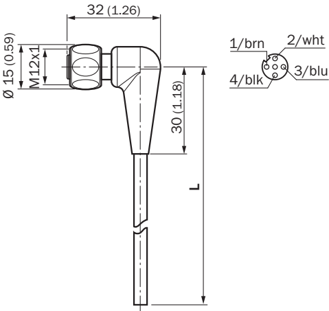
Rysunek wymiarowy (Wymiary w mm)
