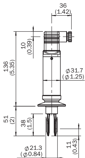
Rysunek wymiarowy
