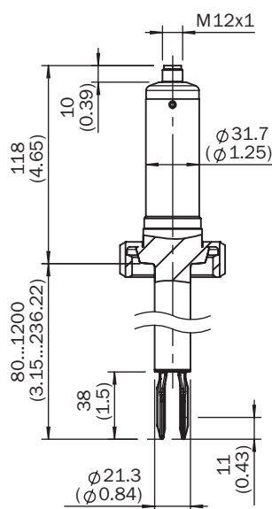
Rysunek wymiarowy
