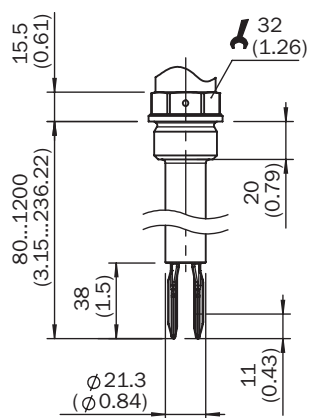
Rysunek wymiarowy: obudowa
