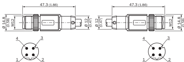
Rysunek wymiarowy (Wymiary w mm)
