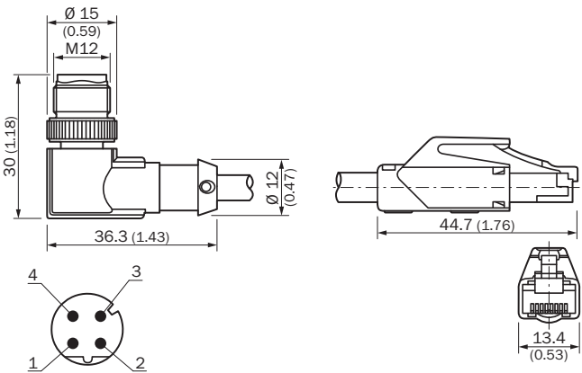
Rysunek wymiarowy (Wymiary w mm)
