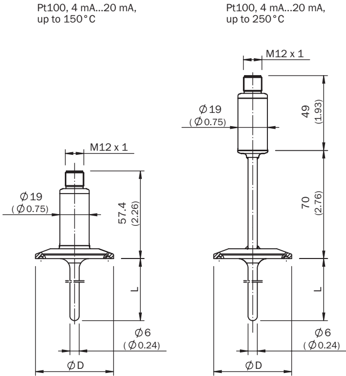
Rysunek wymiarowy
