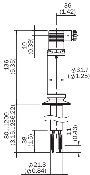
Rysunek wymiarowy
