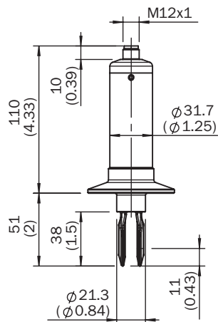
Rysunek wymiarowy
