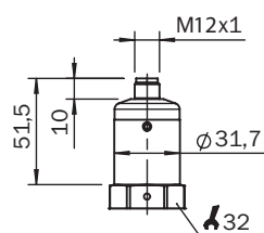
Maßzeichnung Gehäuse
