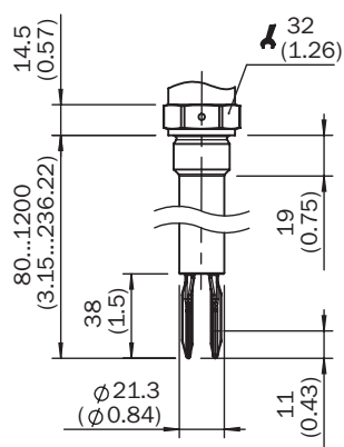
Rysunek wymiarowy: obudowa
