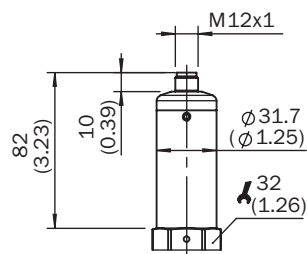
Rysunek wymiarowy: obudowa
