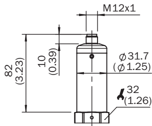
Габаритный чертеж корпуса
