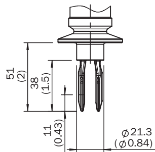
Rysunek wymiarowy: przyłącze procesowe
