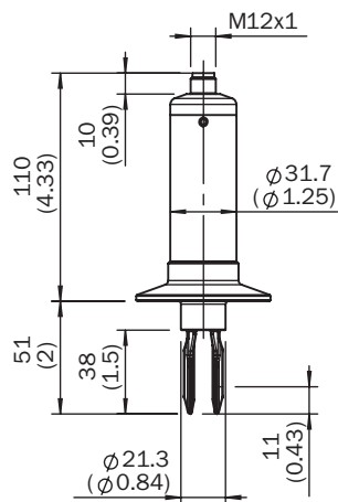
Rysunek wymiarowy: przyłącze procesowe
