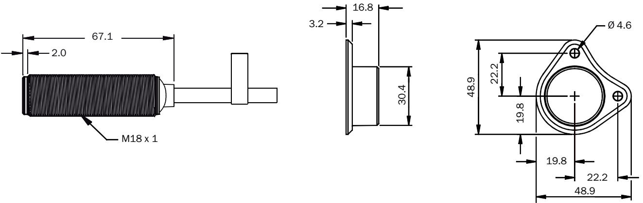
Габаритный чертеж (Размеры, мм)
