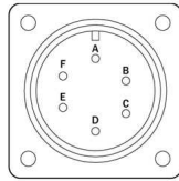
6 Pin MS3102R
