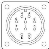
10 Pin MS3102R
